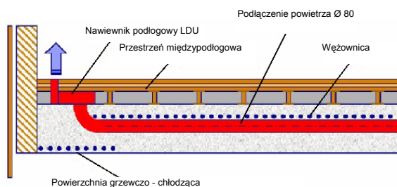
Sposób działania we współpracy ze stropem chłodzącym.
