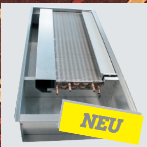
Bodeninduktionsgerät Typ HFB
